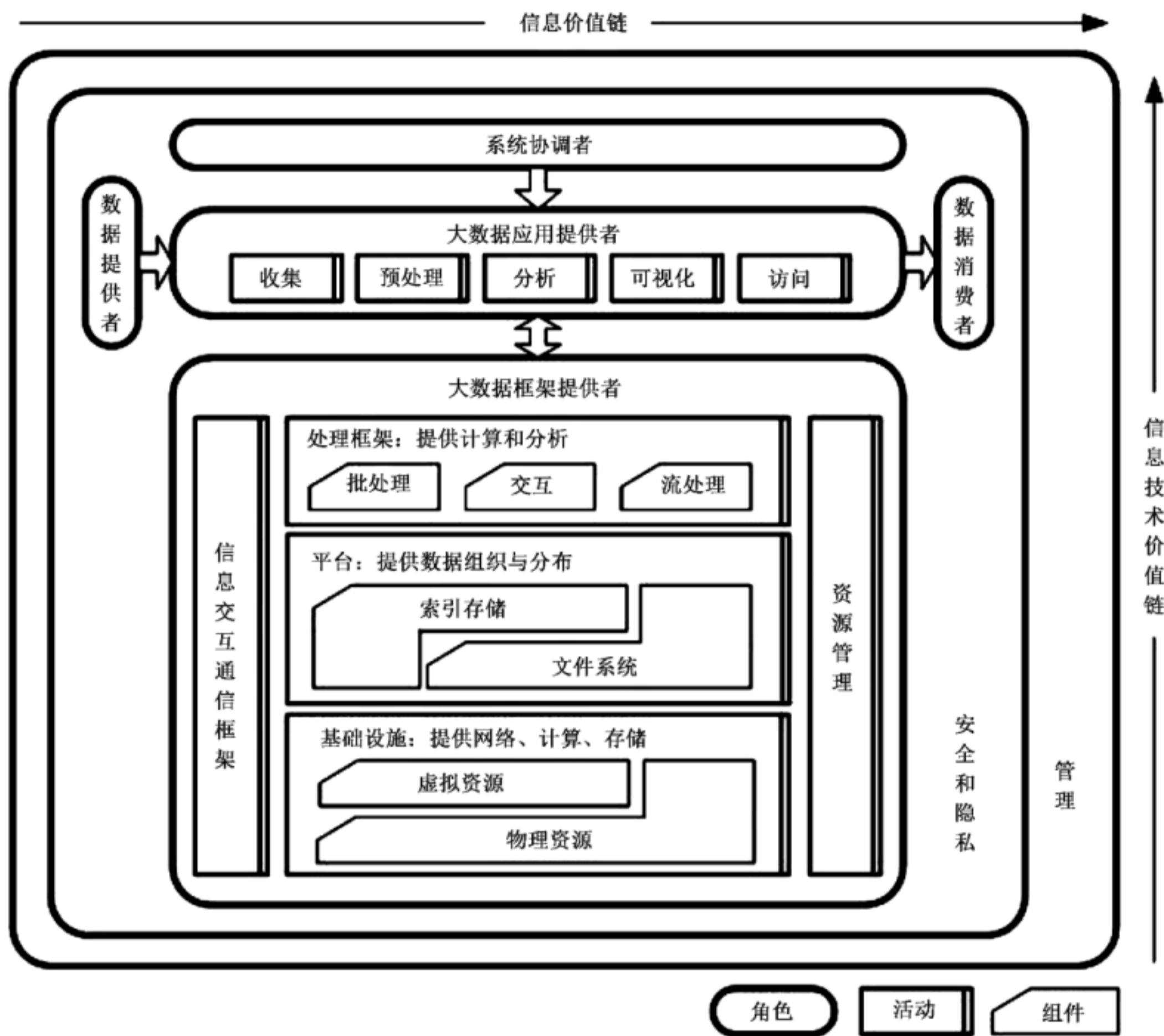
图 1 大数据参考架构
